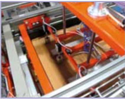
Détail du système de layerpad/tray.
